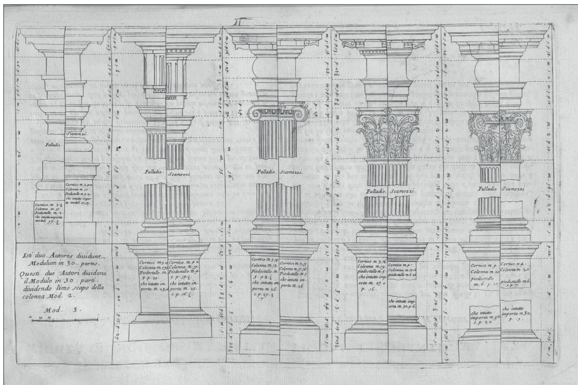
FIGURA 1. ÓRDENES ARQUITECTÓNICOS ESQUEMATIZADOS SEGÚN PALLADIO Y SCAMOZZI. POZZO 1693, SEGUNDO ESTADO. KOMAREK, ROMA. HTTP://WWW.E-RARA.CH/ZUT/CONTENT/PAGEVIEW/1285726 .
