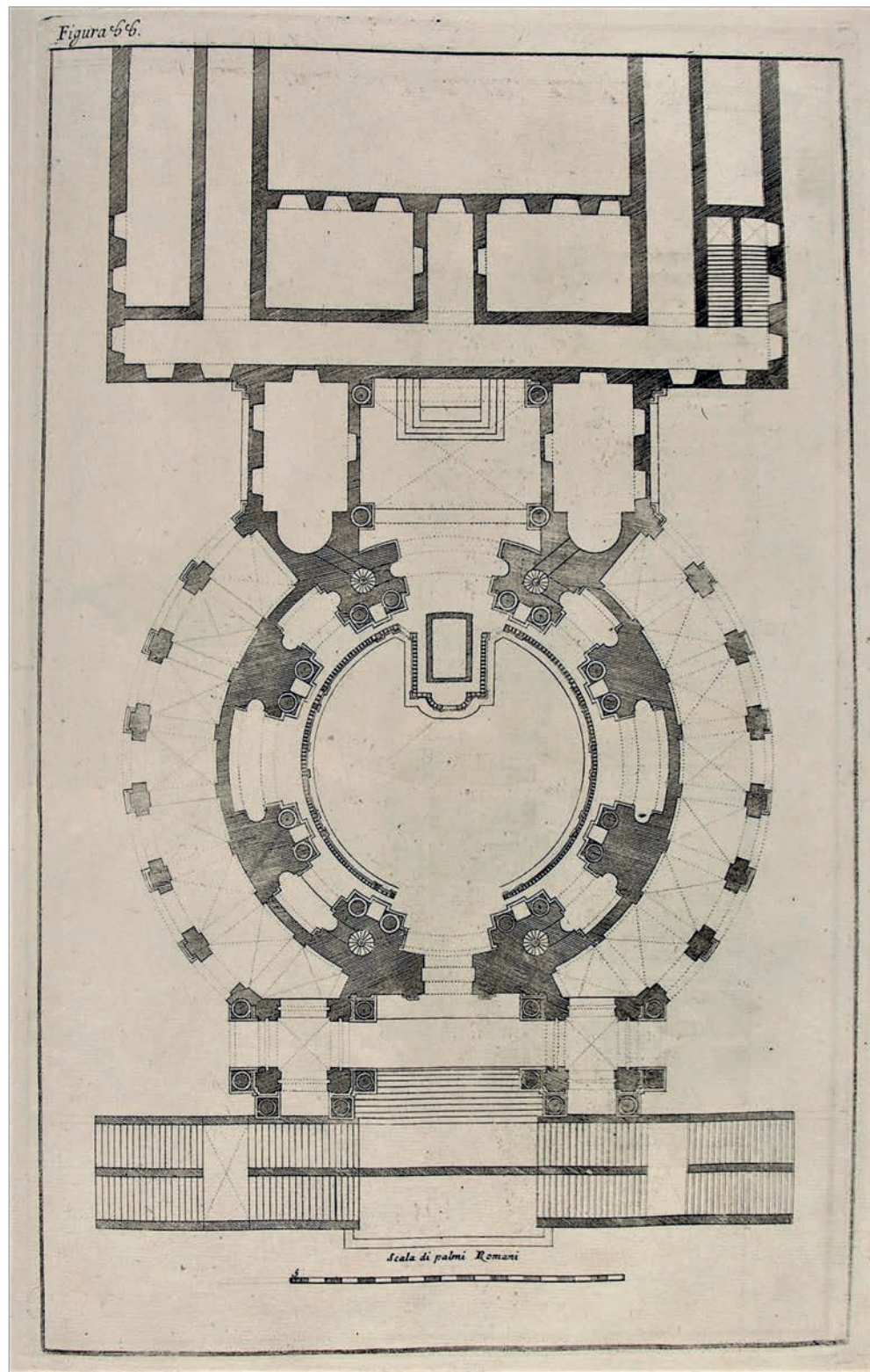
FIGURA 7. POZZO, ANDREA: PERSPECTIVA PICTORUM ARCHITECTORUM. PARS SECONDA , (ROMA 1700). ROMA, JOANNEM GENEROSUM SALOMONI, 1758, FIG. 66.
